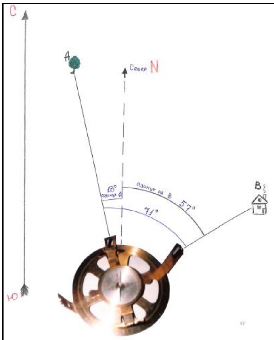
Схема угловых измерений и снятия азимута
