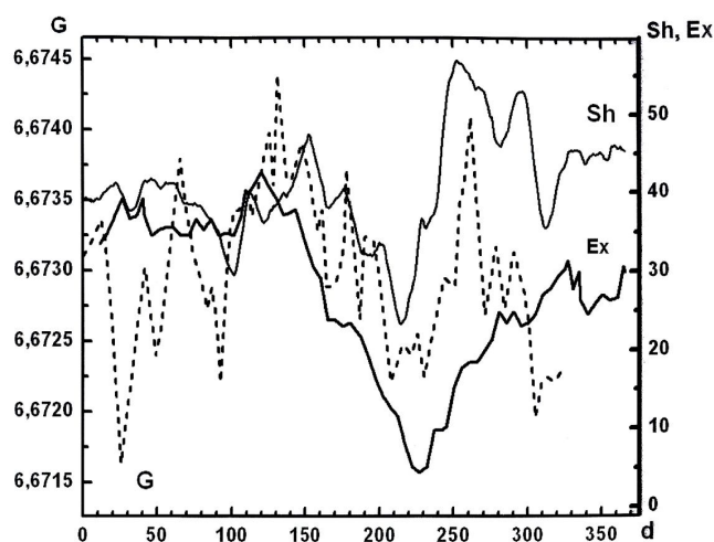
Рис. 8. Сопоставление регистрируемого показателя шторм-гласа (Sh) и артефактных вариаций гравитационной постоянной (G), измеряемой с помощью крутильного маятника на установке В.П. Измайлова – О.В. Карагюза (Москва). Усредненный годовой ход (данные относятся к различным интервалам времени)
